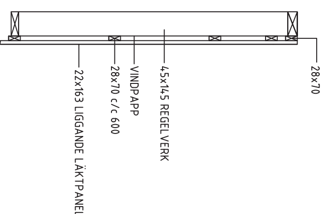
VÄGG SEKTION
